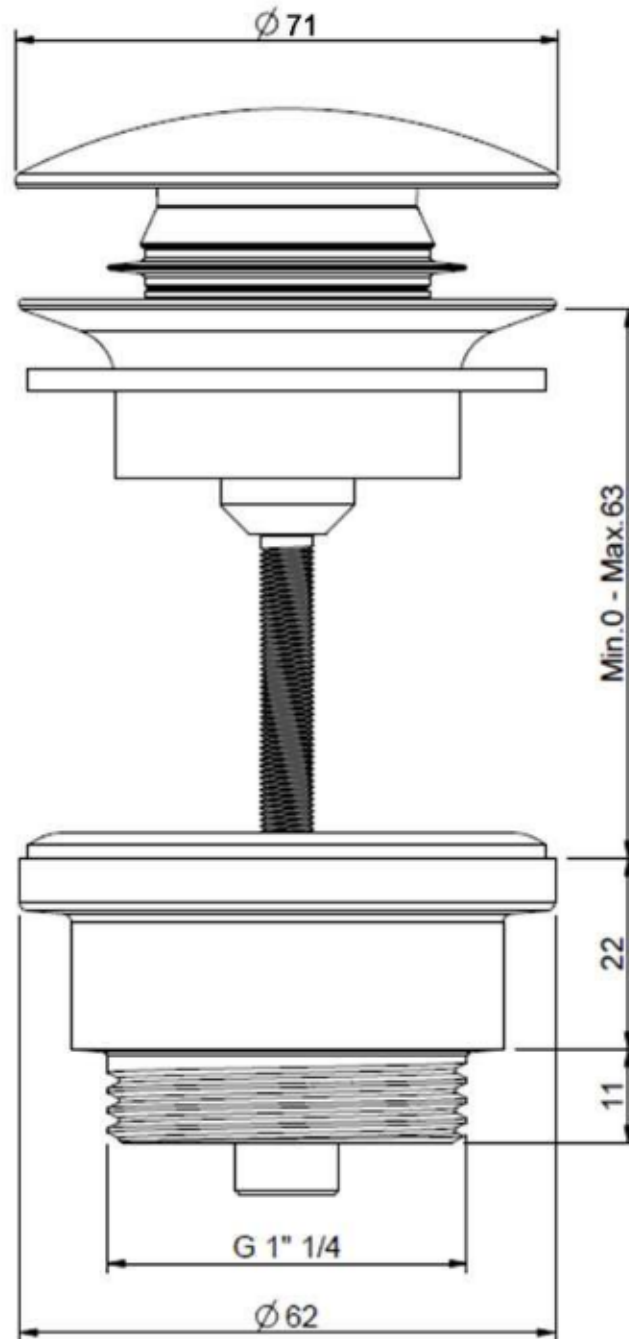
piletta con sistema click clack
